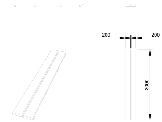
SYSTÉM ROHOŽÍ, FOŠNA TL.50MM NA HRANOLU 50X50MM, SPOJENO HŘEBÍKEM.
